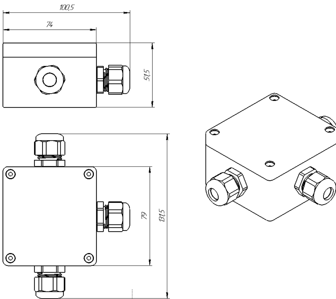
Рисунок А.1 – Габаритные и установочные размеры разветвителя интерфейса RS-422/485 ПР-3УМ
