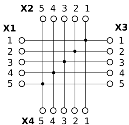
Рисунок А.2 – Схема принципиальная
