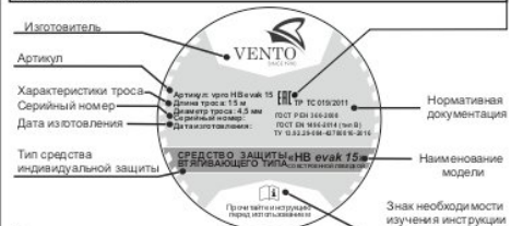
Рис. 2. Маркировка изделия
