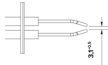
Рисунок 2.1 — Рекомендуемый зазор между электродами зажигания
