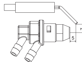
Рисунок 3 — Рекомендуемый зазор между форсункой и электродами зажигания
