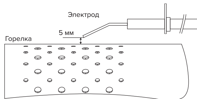
Рисунок 5 — Проверка величины зазора между электродом и горелкой
