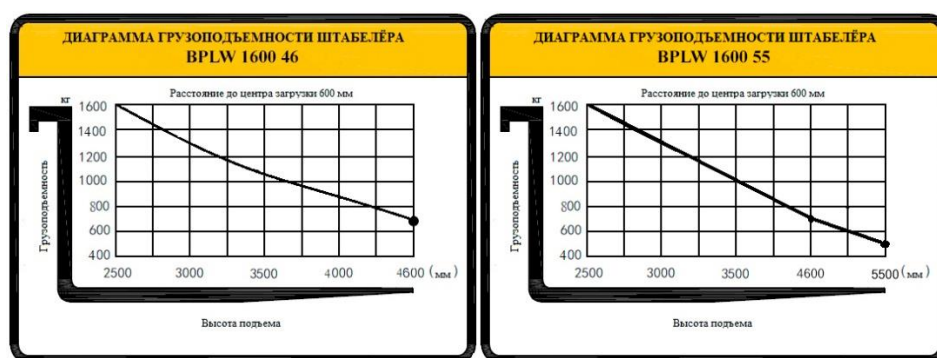
Рисунок. 4 Основные параметры штабелера.
