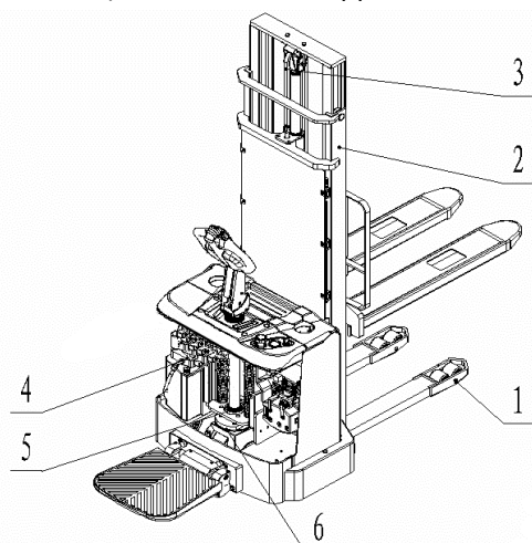
Рисунок. 13 Основные точки смазки.
