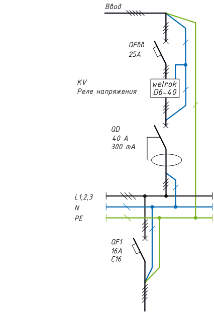
Схема 2. Вариант электрической схемы с трехфазной нагрузкой
