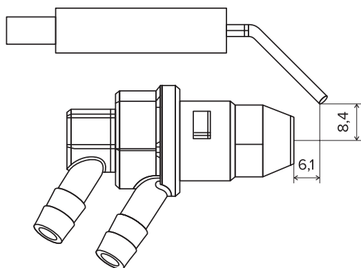
Рисунок 2 — Рекомендуемый зазор между электродами зажигания
