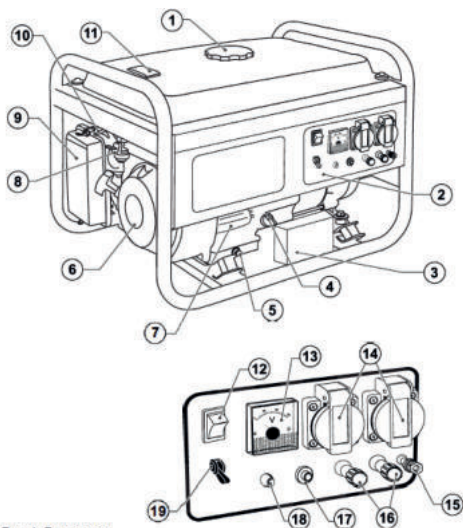
Рис. 1. Генератор
