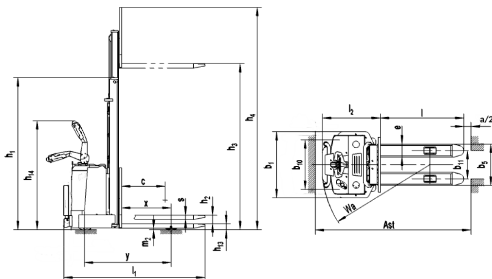
Рисунок. 4 Основные параметры штабелера.
