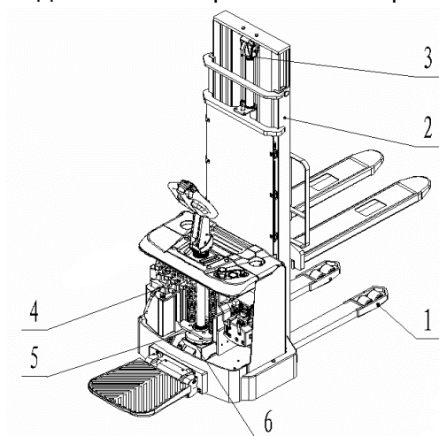
Рисунок. 13 Основные точки смазки.
