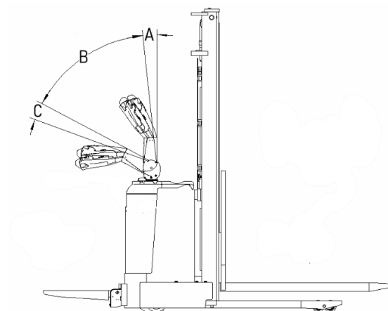
Рисунок 10. Положение румпеля управления.
