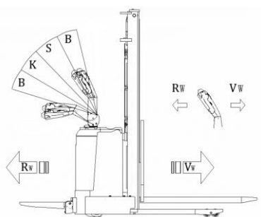
Рисунок 6. Положение румпеля управления.
