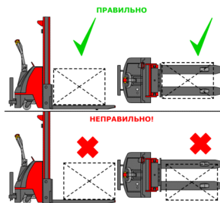
Рисунок 7. Схема расположения груза на вилках.
