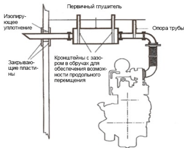
Рис. 5.5.3.1. Система выхлопа
