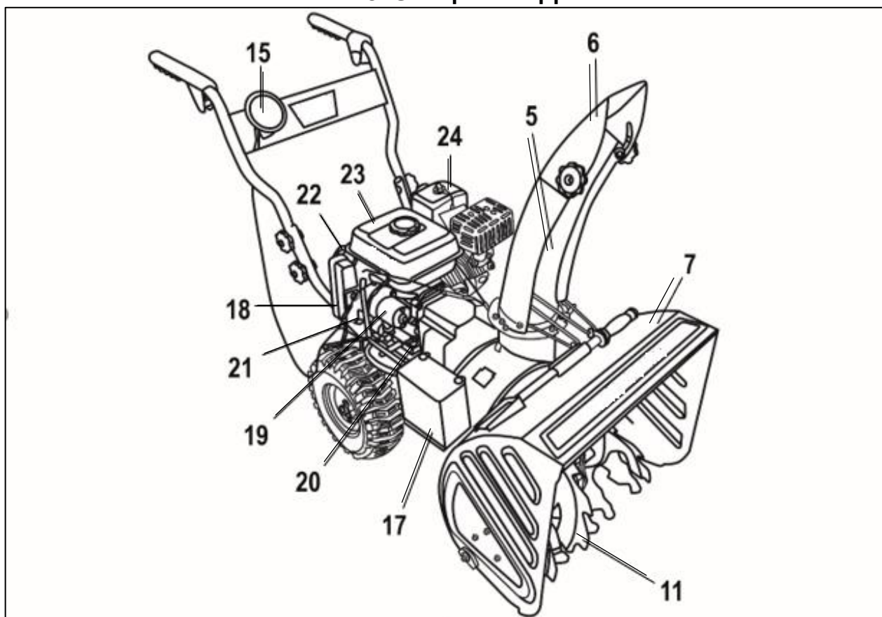
Рис. 1. Общий вид
