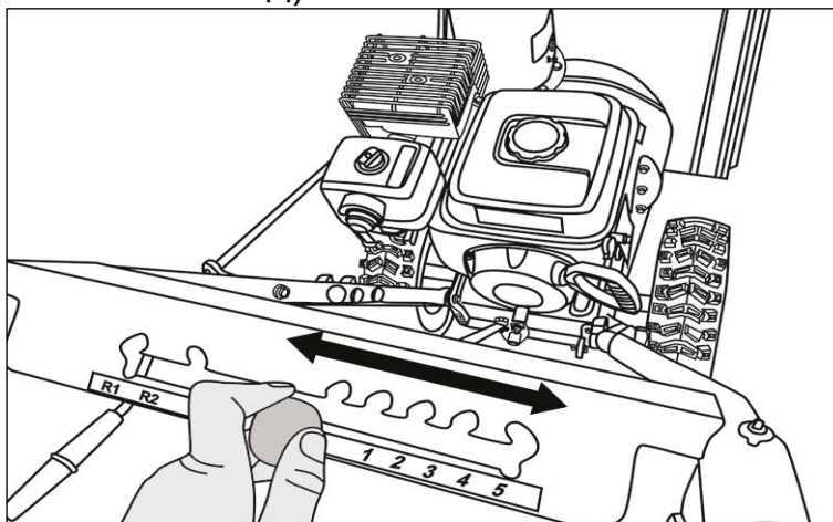
Рис. 42. Включение скорости
