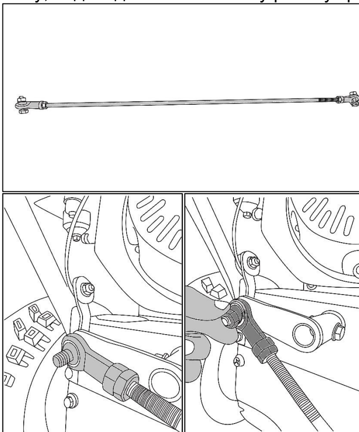
Рис. 17. Установка тяги
