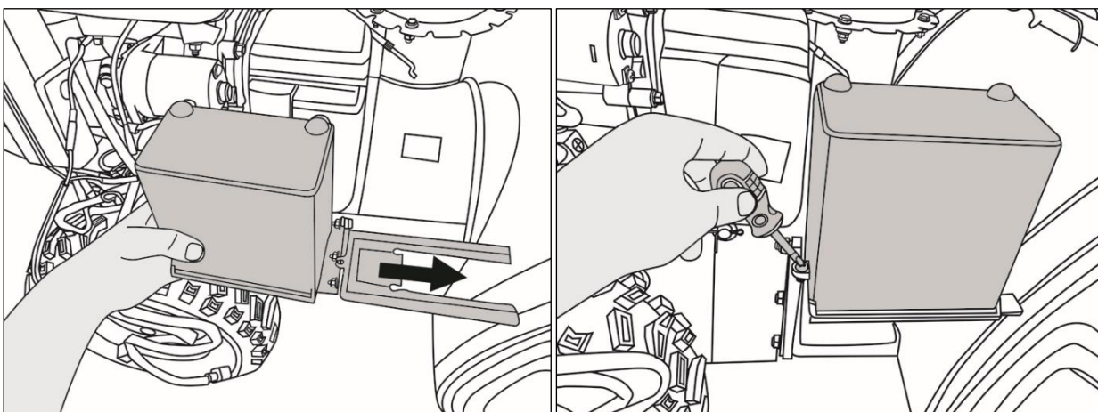
Рис. 26. Установка подключенного аккумулятора на раму
