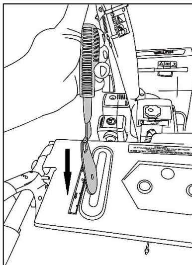
Рис. 9. Установка рукоятки
