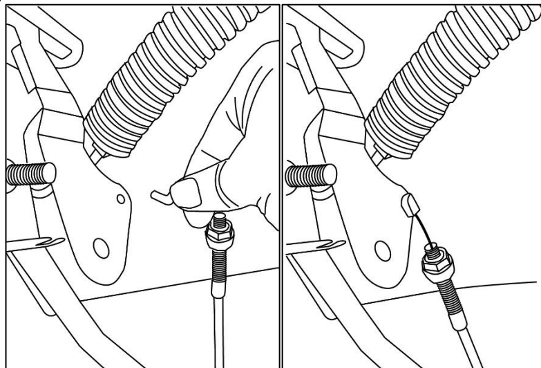
Рис. 10. Установка тросика
