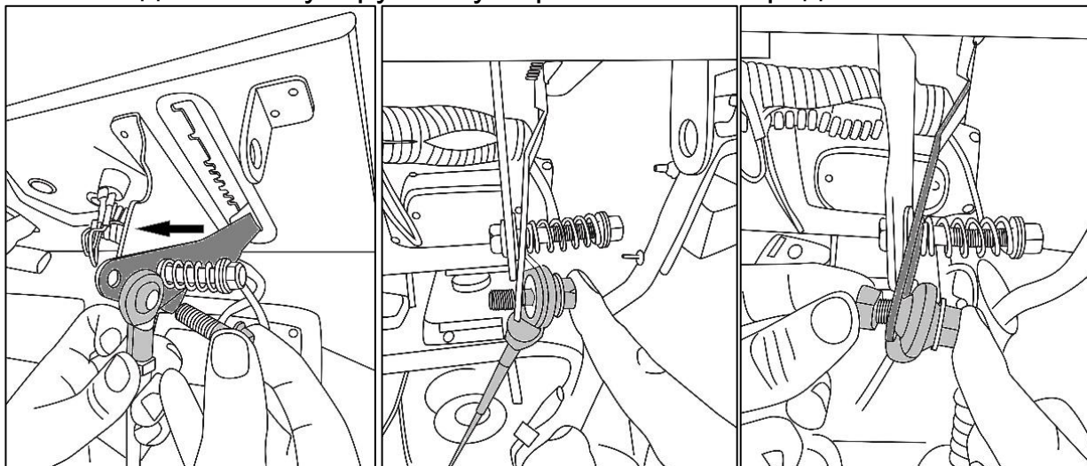
Рис. 18. Установка тяги
