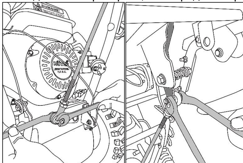
Рис. 19. Установка тяги
