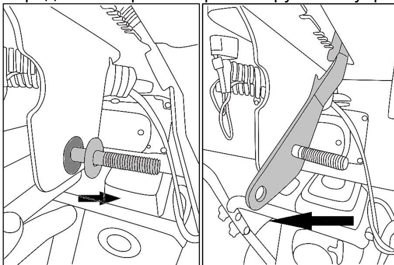
Рис. 15. Установка рукоятки
