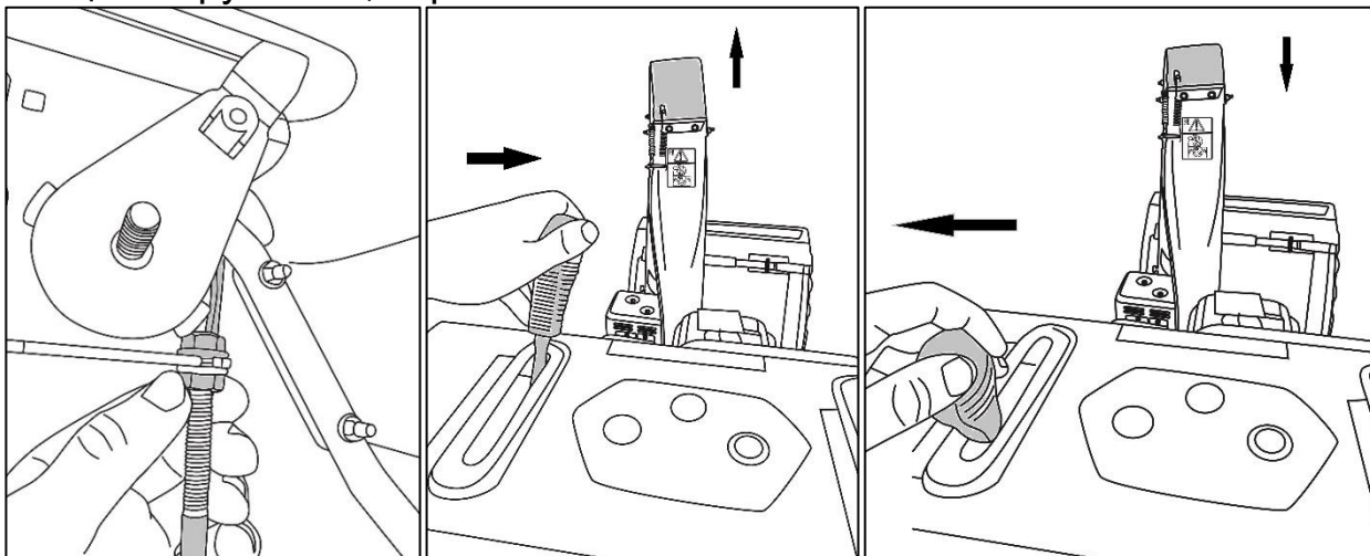
Рис. 13. Регулировка тросика
