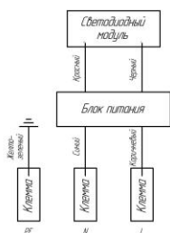
Схема электрическая соединений
