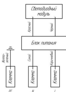
Схема электрическая соединений
