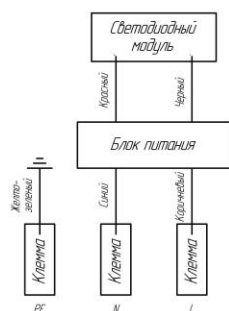
Схема электрическая соединений
