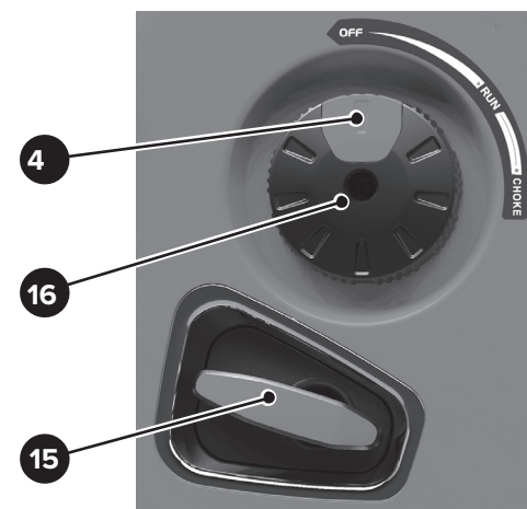
Рисунок 7 — Элементы управления запуском двигателя
