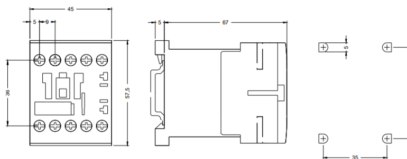
Рис.6 Габаритные размеры 3RT1015, 3RT1016, 3RT1017 с 3RH1911-1FA
