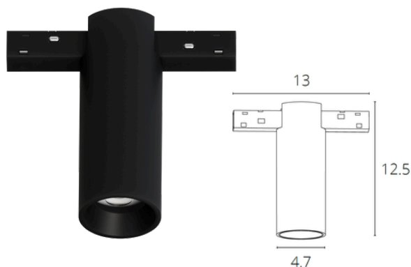
A7269PL-1BK A7269PL-1WH LED | 8W | 830Lm | 4000K
