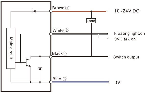
NPN Output
