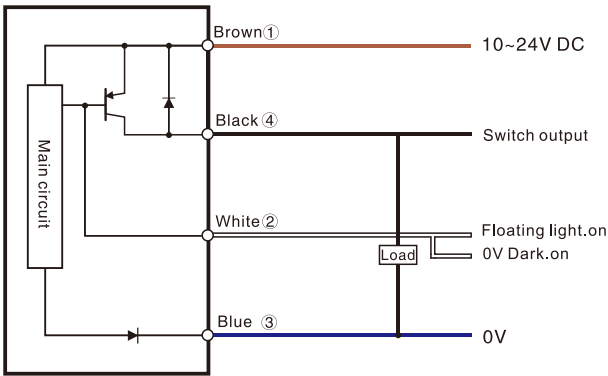
PNP Output
