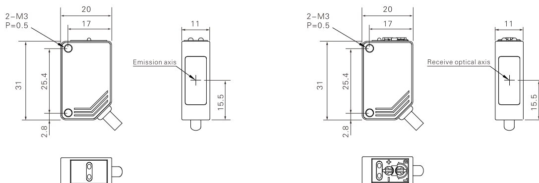
ELE-TM30N/P
