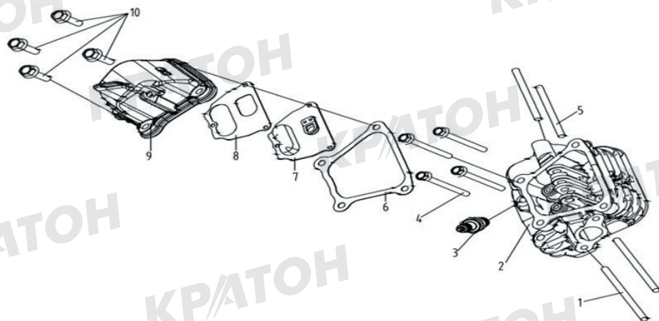
Схема сборки № 1
