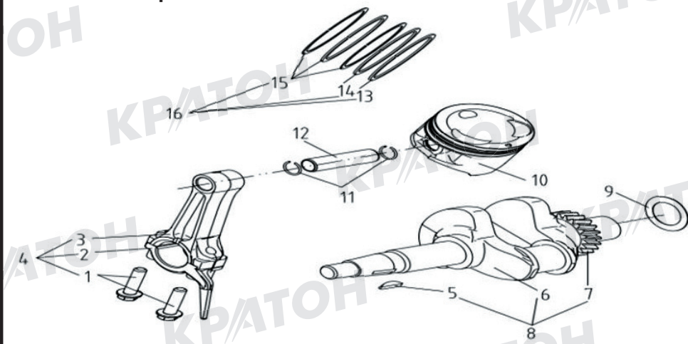
Схема сборки № 4
