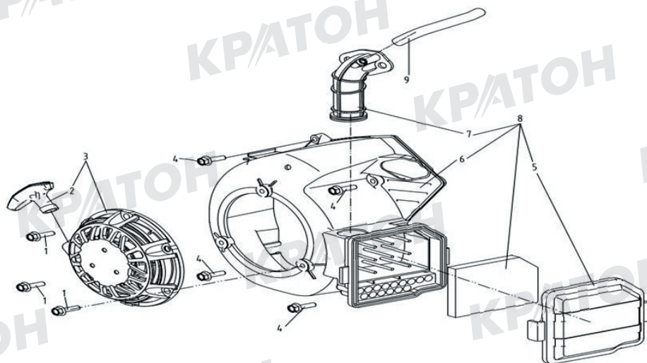
Схема сборки № 6
