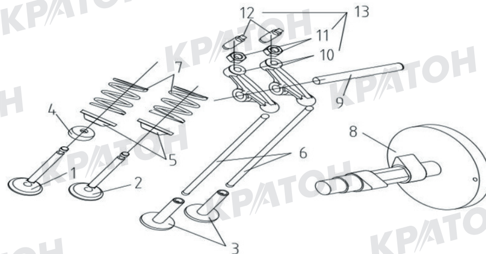
Схема сборки № 7
