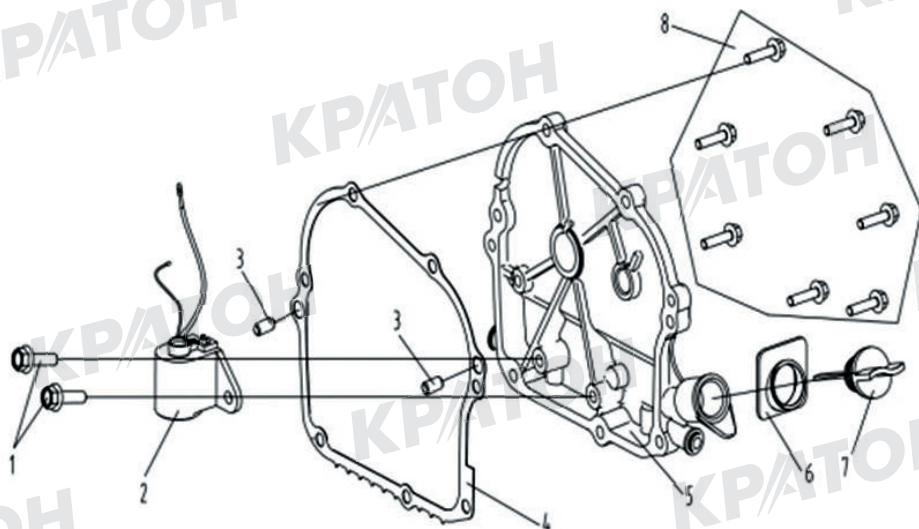
Схема сборки № 3
