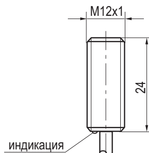
Габаритный чертеж
