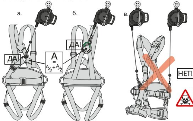
Рис. 3. Соединение «НВ evak» с привязью
