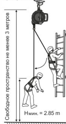
Рис. 4. Запас свободного пространства
