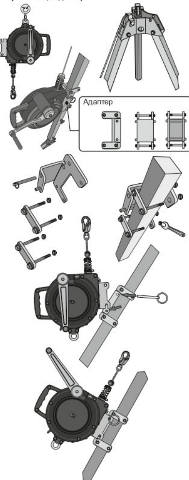
Рис. 7. Способы установки «НВ evak» на треногу при помощи адаптера
