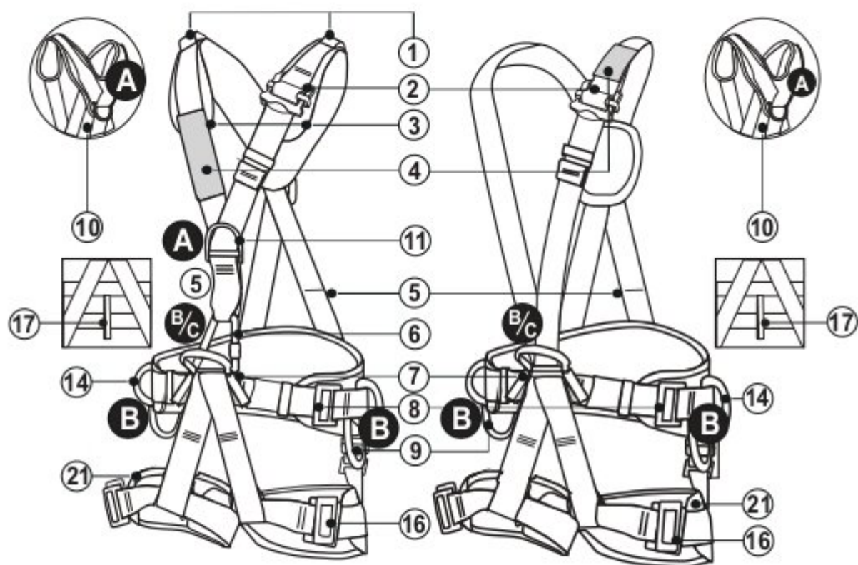
Рис. 1. Внешний вид и составные части привязей (список составных частей см. на стр. 18-19)
