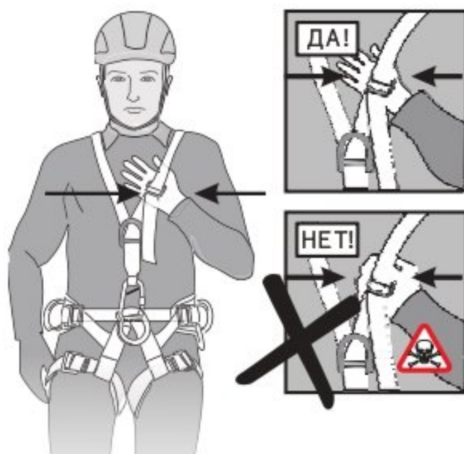
Рис. 8. Натяжение лямок привязи
