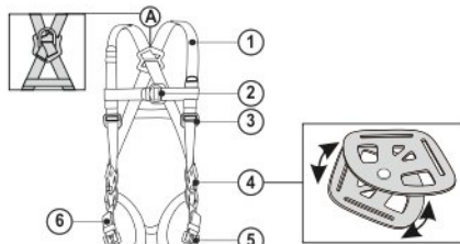
Рис. 1. Внешний вид и состав привязи
