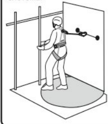
Рис. 11. Способ организации удерживающей системы
