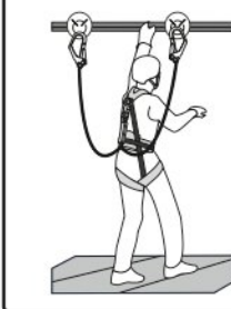
Рис. 10. Страховочная система
