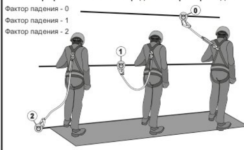
Рис. 10. Страховочная система
