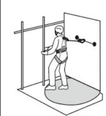
Рис. 9. Способ организации удерживающей системы
