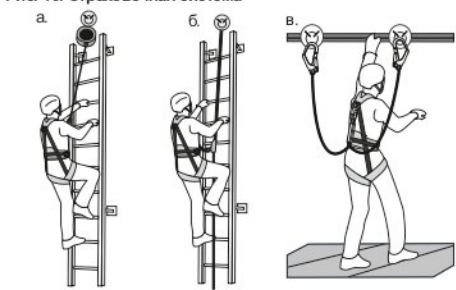
Рис. 10. Страховочная система
