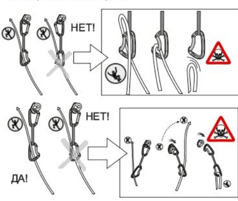
Рис. 7. Прощелкивание веревки
