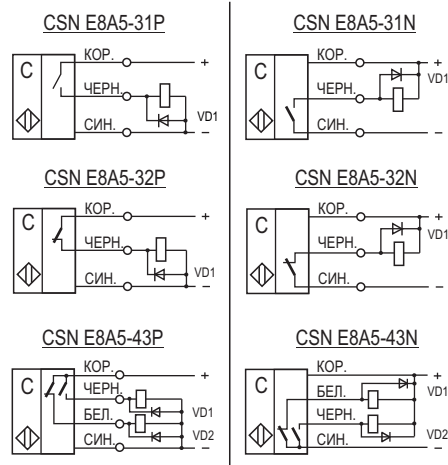
Схемы подключения
