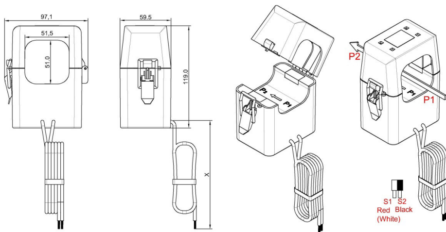
Рисунок 3.10 – Внешний вид и размеры ТРП-0,66-3/50
