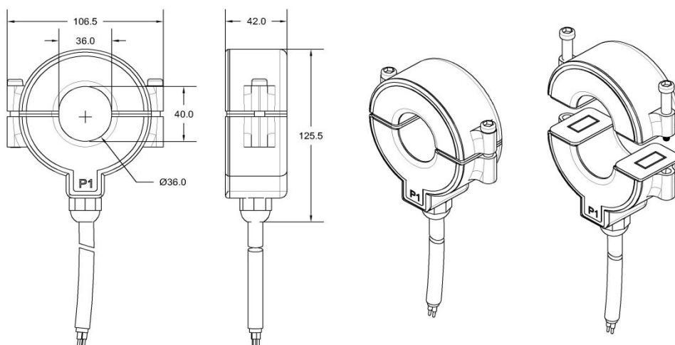
Рисунок 3.1 – Внешний вид и размеры ТРП-0,66-1/36
