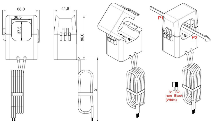
Рисунок 3.9 – Внешний вид и размеры ТРП-0,66-3/36
