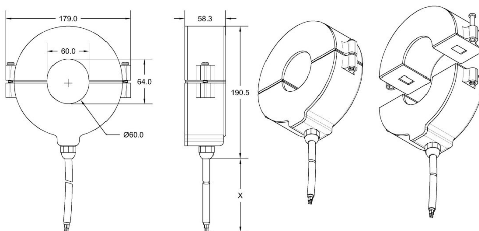
Рисунок 3.1 – Внешний вид и размеры ТРП-0,66-1/36
