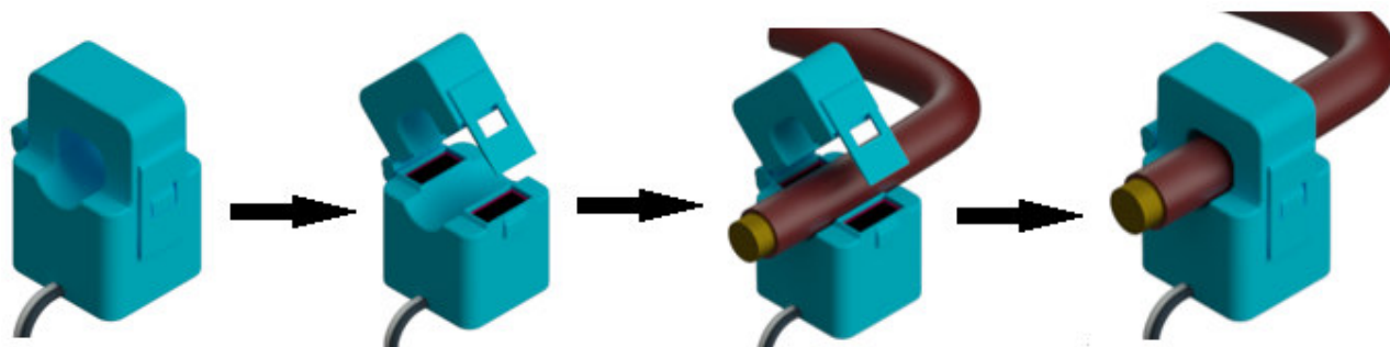
Рисунок 3.12 – Вариант установки для ТРП-0,66-3/16, ТРП-0,66-3/24, ТРП-0,66-3/36, ТРП-0,66-3/50
