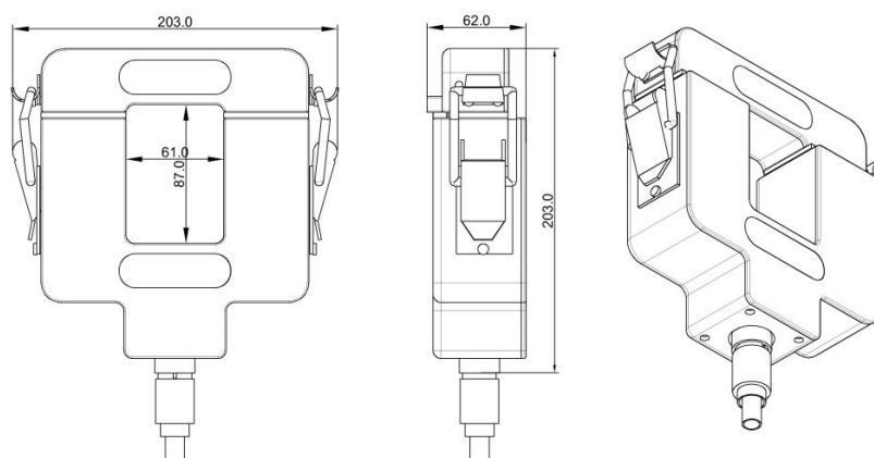
Рисунок 3.5 – Внешний вид и размеры ТРП-0,66-2/68
