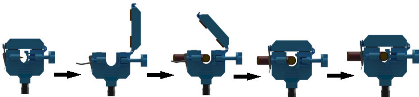
Рисунок 3.13 – Вариант установки для ТРП-0,66-2/30, ТРП-0,66-2/40, ТРП-0,66-2/68, ТРП-0,66-2/162
