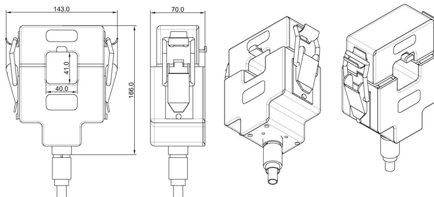
Рисунок 3.4 – Внешний вид и размеры ТРП-0,66-2/40
