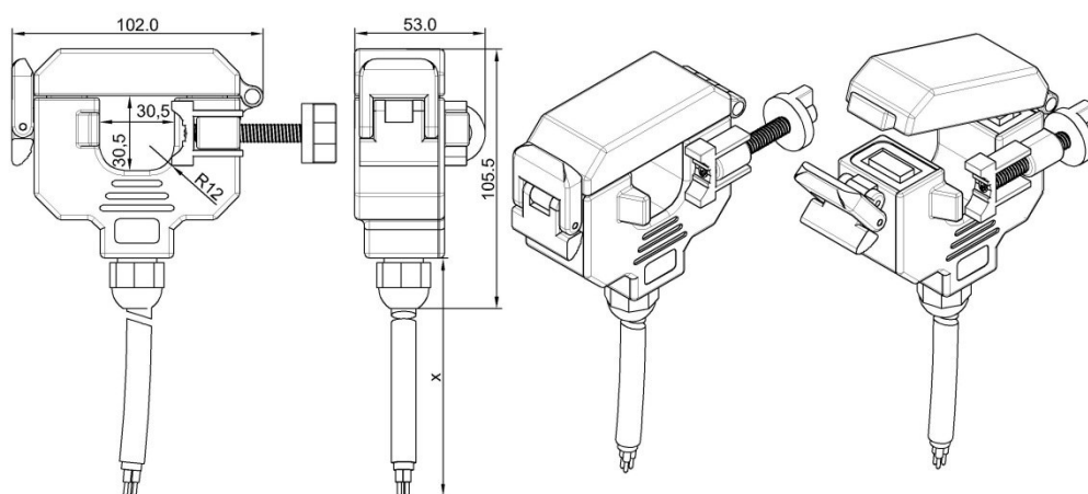
Рисунок 3.3 – Внешний вид и размеры ТРП-0,66-2/30
