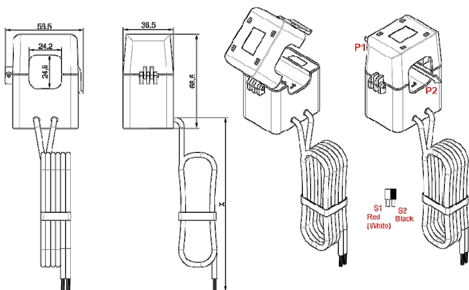
Рисунок 3.8 – Внешний вид и размеры ТРП-0,66-3/24
