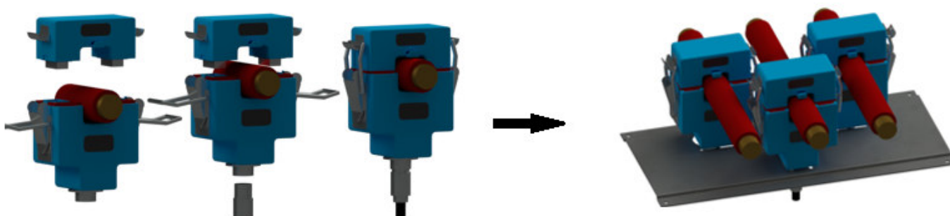
Рисунок 3.15 – Вариант крепления трансформаторов на металлической пластине.
