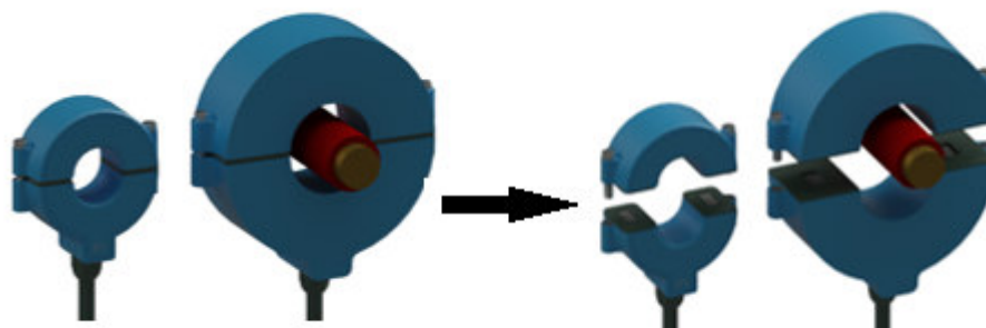
Рисунок 3.14 – Вариант установки для ТРП-0,66-1/36, ТРП-0,66-1/60
