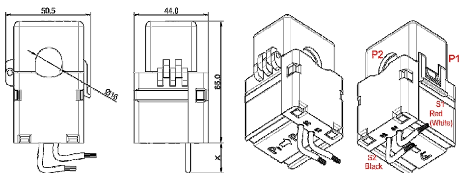
Рисунок 3.7 – Внешний вид и размеры ТРП-0,66-3/16
