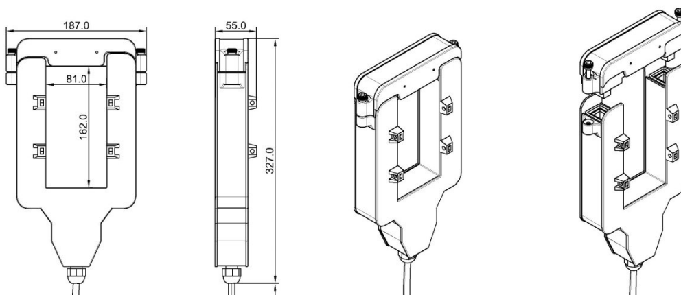
Рисунок 3.6 – Внешний вид и размеры ТРП-0,66-2/162
