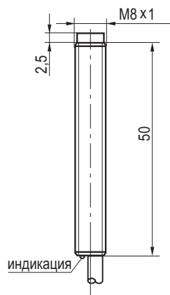
Габаритный чертеж
