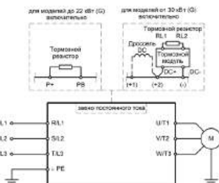
Рис. 3.2.4 Подключение силовых клемм
