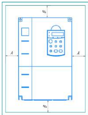
Рис. 3.1 - Рекомендуемые расстояния при монтаже
