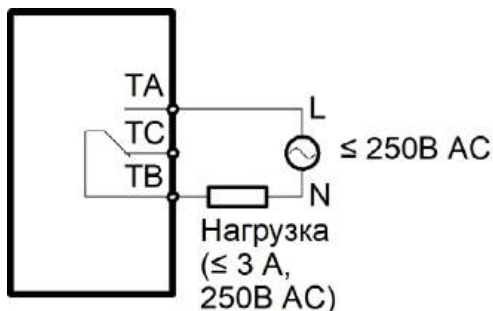
Рис. 3.10 – Схема подключения нагрузки переменного тока к релейному выходу
