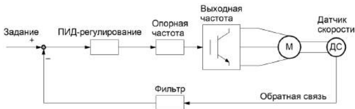
Рис.6.23 Схема ПИД-регулирования
