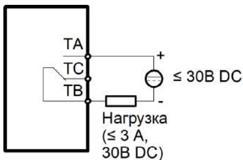
Рис. 3.11 – Схема подключения нагрузки постоянного тока к релейному выходу
