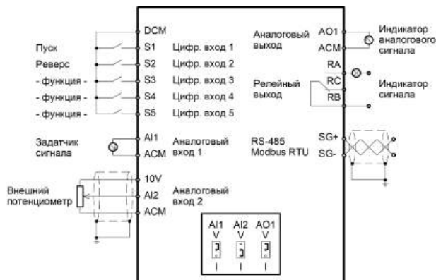
Рис. 3.4а Схема подключения управляющих клемм серии LCI(S)
