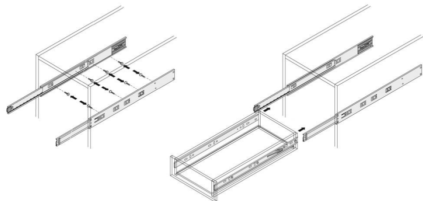
Установка ящика
