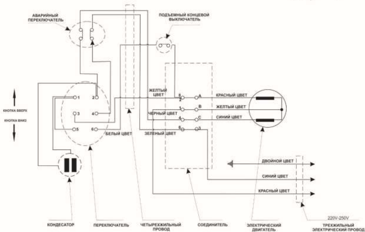
Рисунок 5. Электрическая схема мини тали.
