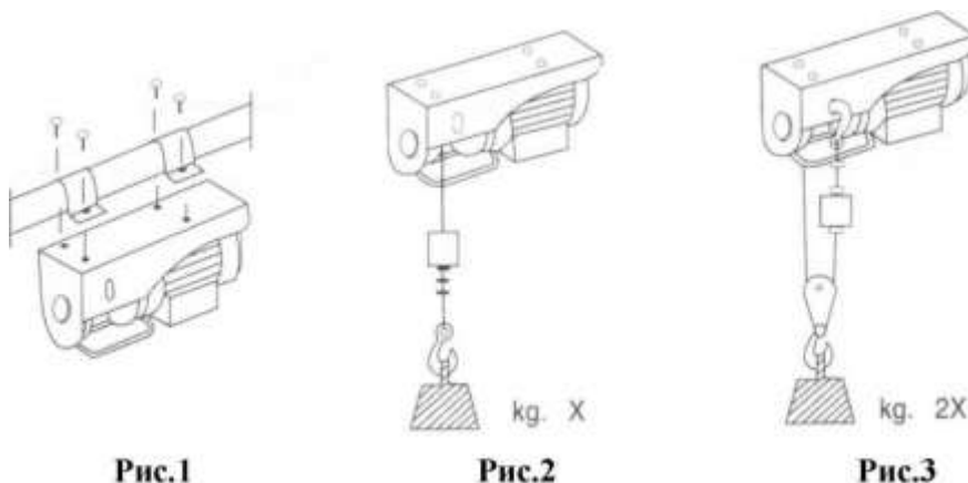
Рисунок 1. Установка мини тали.
