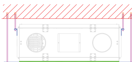
Вид слева
