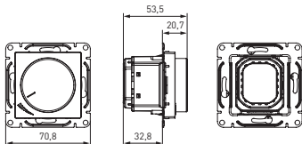
Рис. 1 Механизм светорегулятора UP1-D*-00
