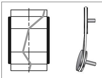
Abb 8 Darstellung einer Kombination aller drei Fehlausrichtungen
