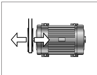
图14 水平方向的角度对中调节
