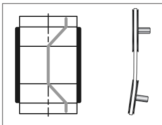
图6 显示水平方向的角度不对中
