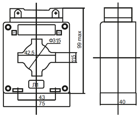
Рис. 4 Габаритные и установочные размеры трансформаторов тока ТСП-0,66-40
