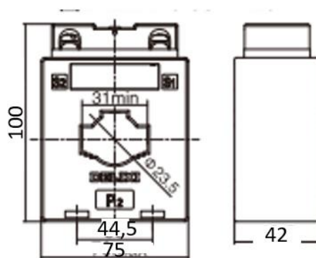
Рис. 2 Габаритные и установочные размеры трансформаторов тока ТШП-0,66-30 0,5
