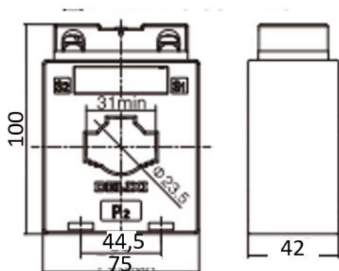
Рис. 3 Габаритные и установочные размеры трансформаторов тока ТСП-0,66-30 0,5S
