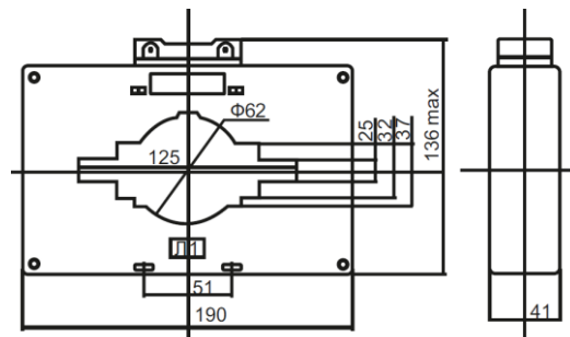
Рис. 8 Габаритные и установочные размеры трансформаторов тока ТСП-0,66-120
