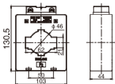
Рис. 5 Габаритные и установочные размеры трансформаторов тока ТСП-0,66-60
