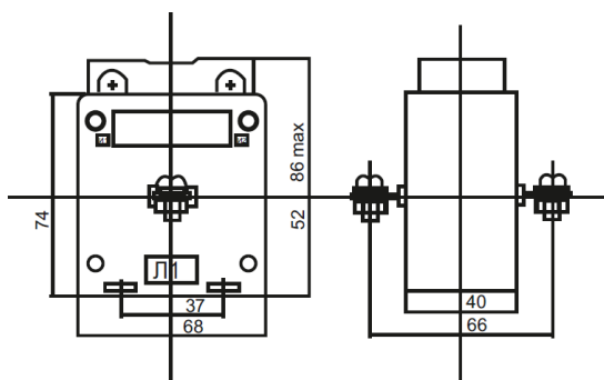
Рис. 1 Габаритные и установочные размеры трансформаторов тока ТОП-0,66
