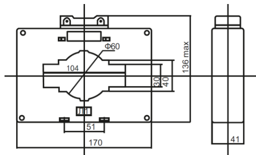
Рис. 7 Габаритные и установочные размеры трансформаторов тока ТСП-0,66-100
