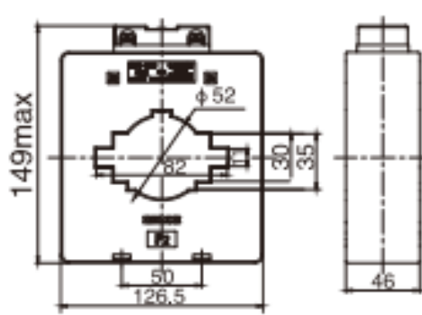
Рис. 6 Габаритные и установочные размеры трансформаторов тока ТСП-0,66-80
