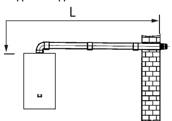
Варианты горизонтальной установки дымохода
