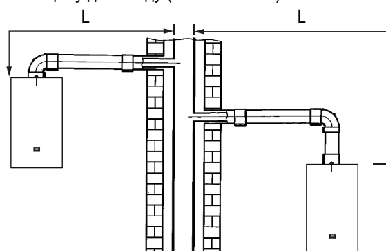
Варианты установки при присоединении к общему дымоходу (LAS - система)
