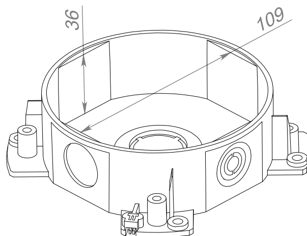
МОНТАЖНАЯ КОРОБКА МК-4, МК-4 ПРО ГАБАРИТНЫЕ И УСТАНОВОЧНЫЕ РАЗМЕРЫ
