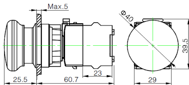
БК30-01МВ/Р/Р, БК30-М11МВ/Р/Р
