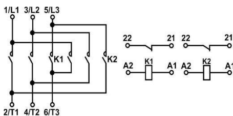
г) реверсивный, вспомогательная цепь 2«р» K1 - контактор «Вперед»; K2 - контактор «Назад»
