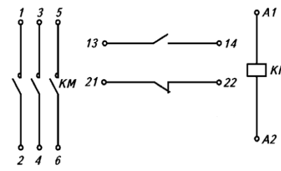
в) вспомогательная цепь 1«з»+1«р»
