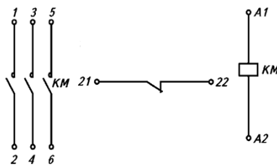
б) вспомогательная цепь 1«р» KM - контактор
