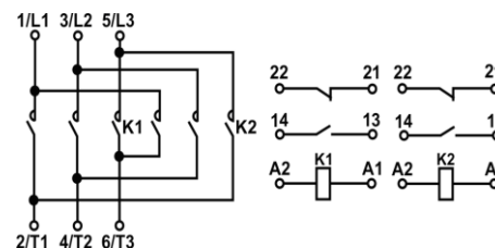
е) реверсивный, вспомогательная цепь 2«р»+2«з» K1 - контактор «Вперед»; K2 - контактор «Назад»
