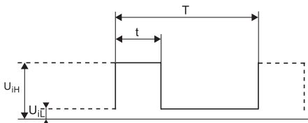
Рис. 17 Иллюстрация ШИМ сигнала
