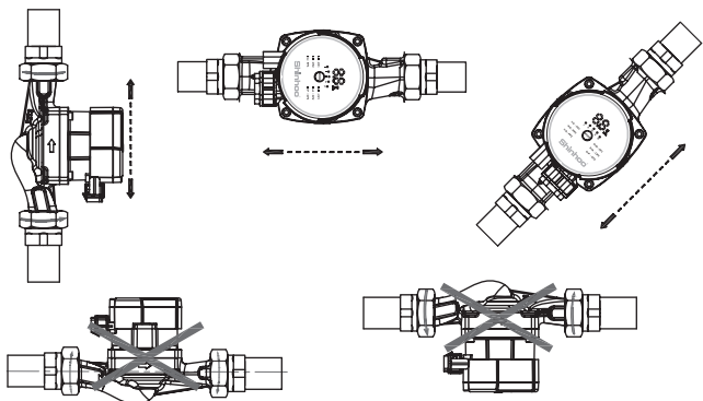
Рис. 5 Расположение насоса
