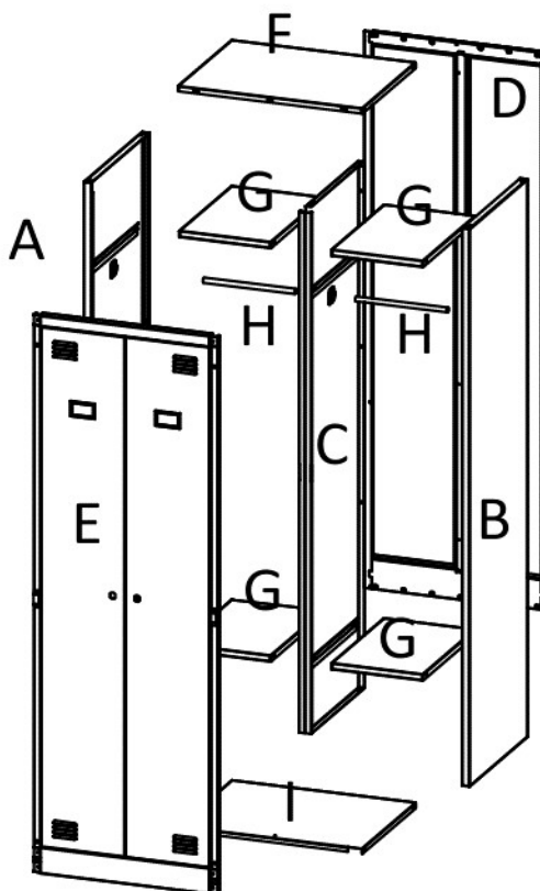
ДЕТАЛИ ШКАФА
