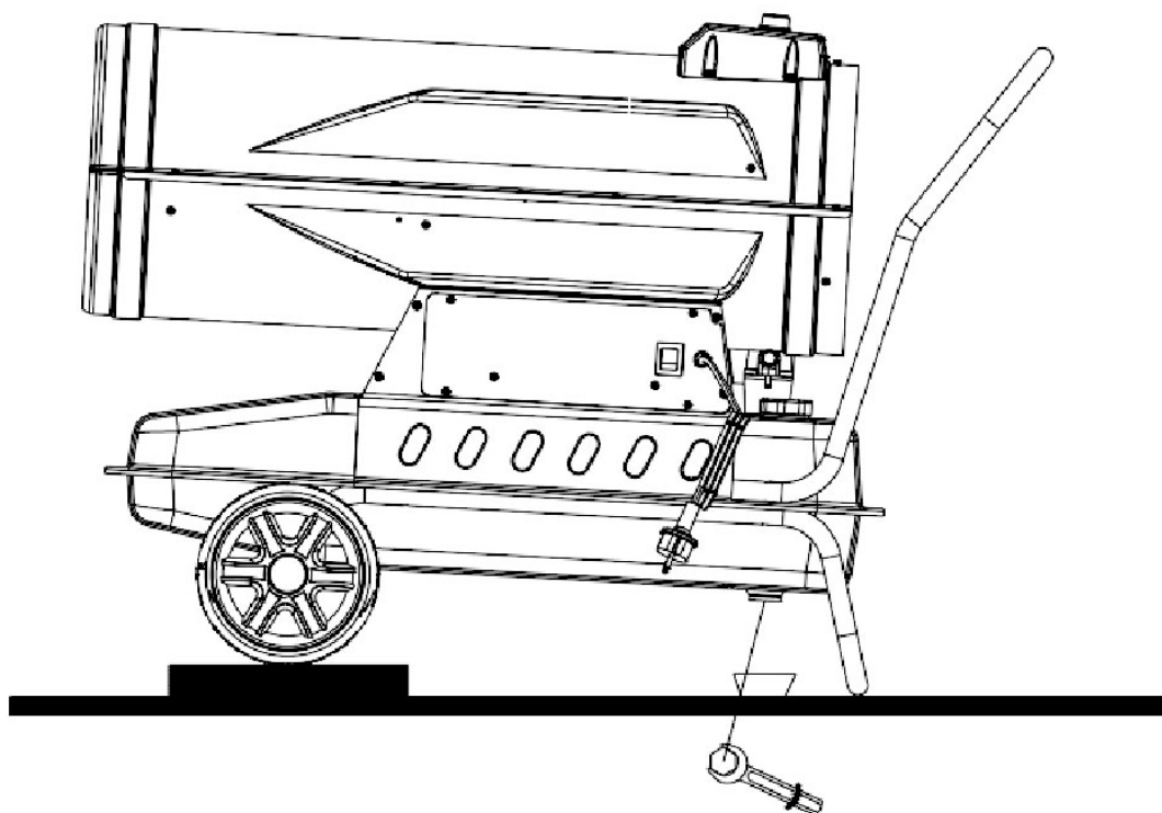
Рисунок 10. Очистка топливного бака
