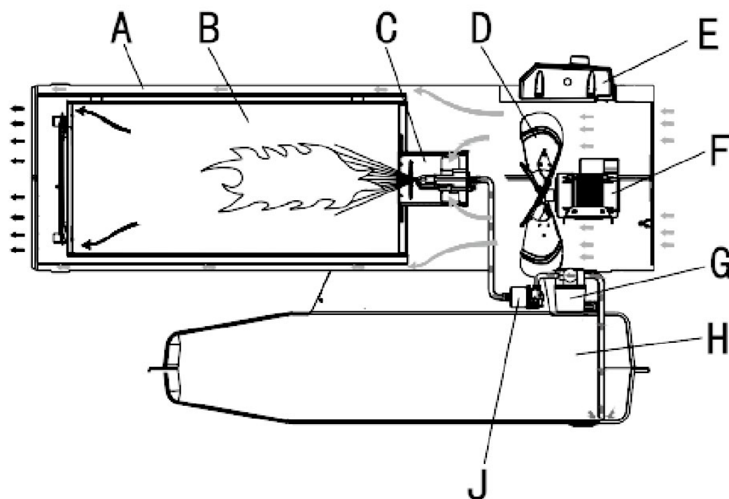
Рисунок 7. Принцип работы Y30, Y50, Y80
