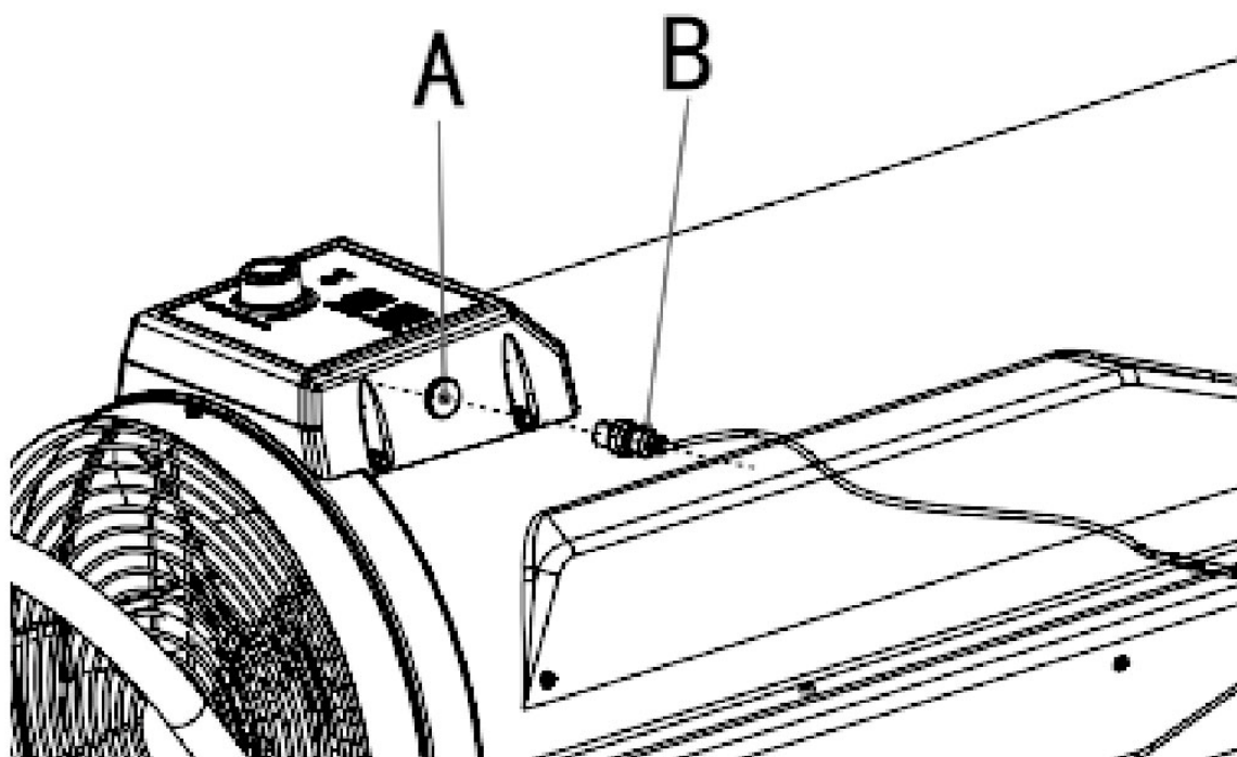
Рисунок 9. Подключение внешнего термостата
