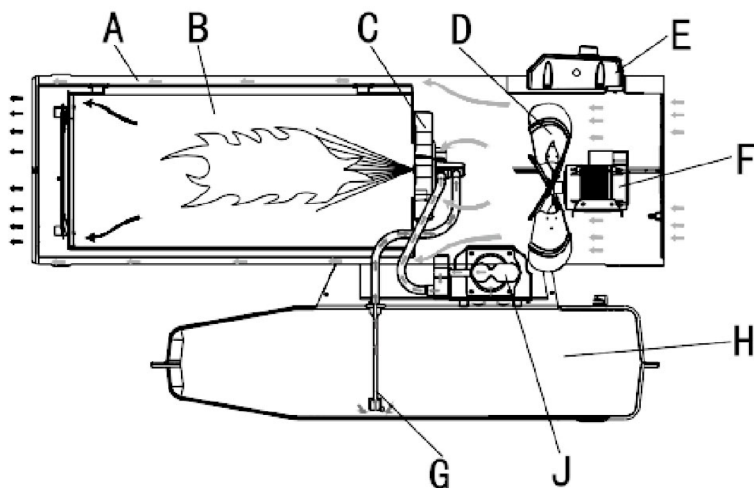
Рисунок 6. Принцип работы Y20
