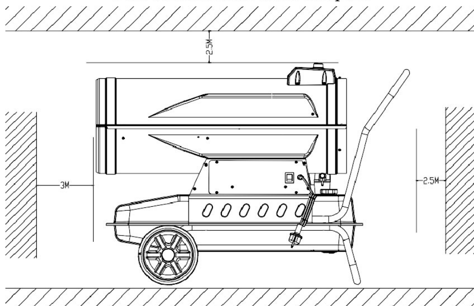
Рис. 2. Расстояние спереди и сзади
