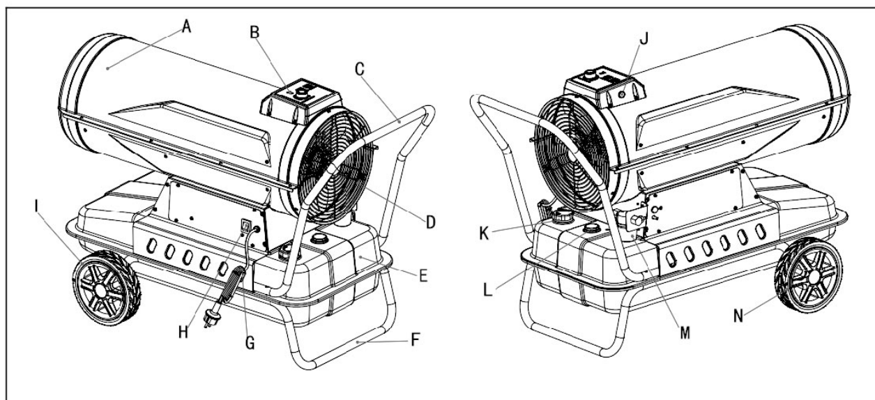
Рисунок 3. Внешний вид устройства и его компоненты
