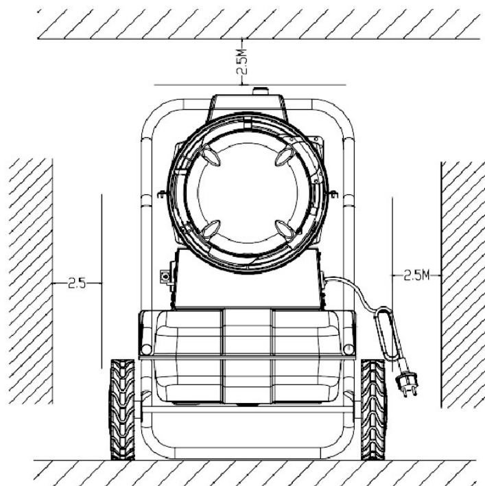
Рис. 1. Расстояние слева и справа
