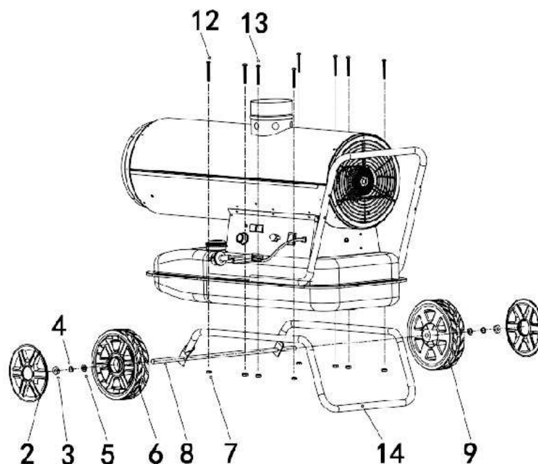
Рис.5 Конструкция
