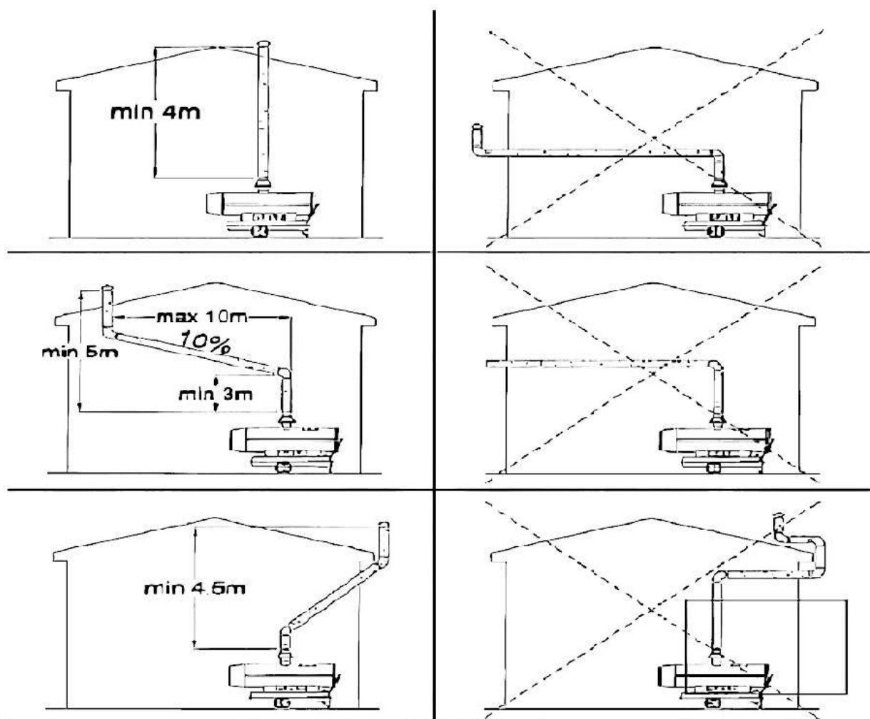
Рис. 9 Подключение внешней трубы отвода выхлопных газов
