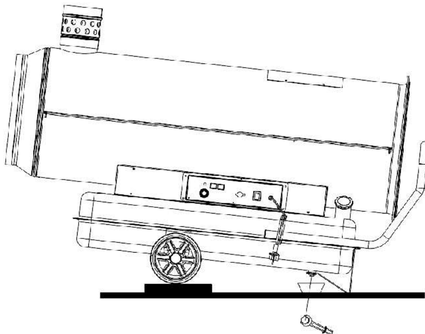
Рис.10 Очистка топливного бака
