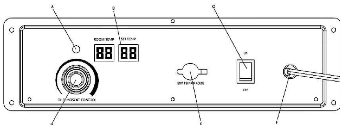
Рис 7. Панель управления
