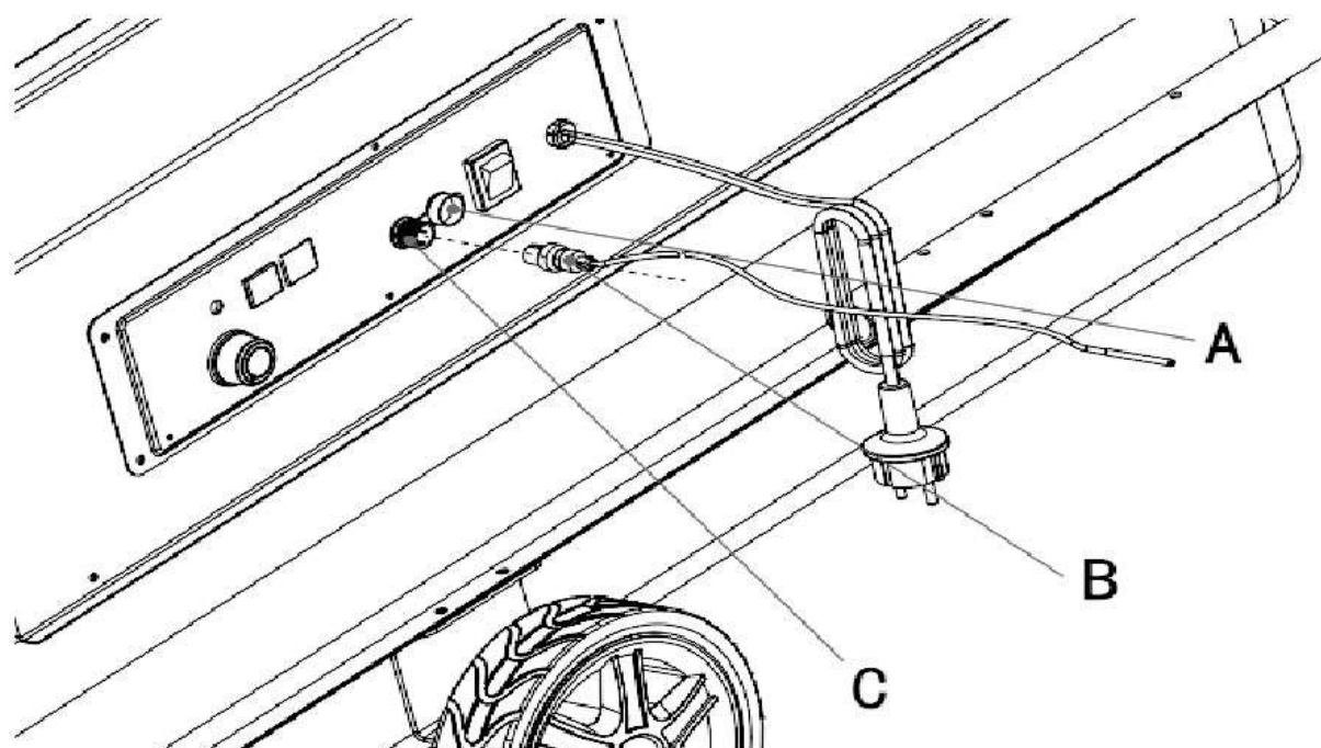
Рис 8 Подключение внешнего термостата
