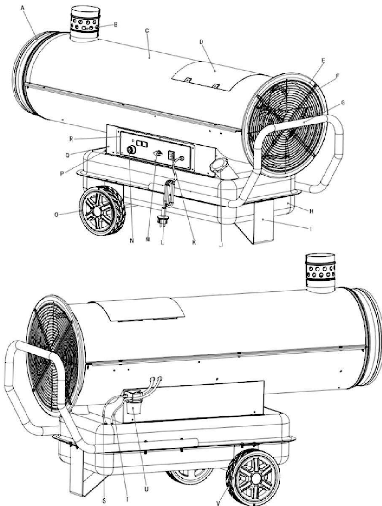
Рисунок 3 Внешний вид оборудования и компоненты
