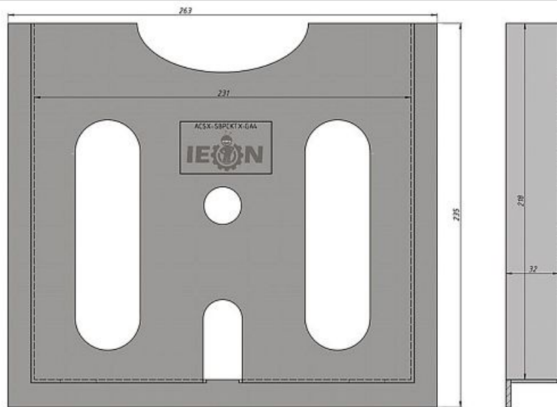
ACSX-SBPCKTX-GA4, чертеж
