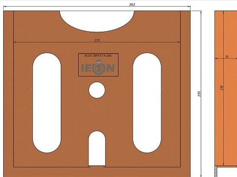
ACSX-SBPCKTX-OA4, чертеж
