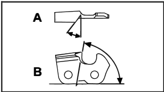
A = угол заточки B = угол боковой пластины
