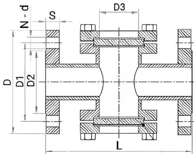
Рисунок 2 - Размеры
