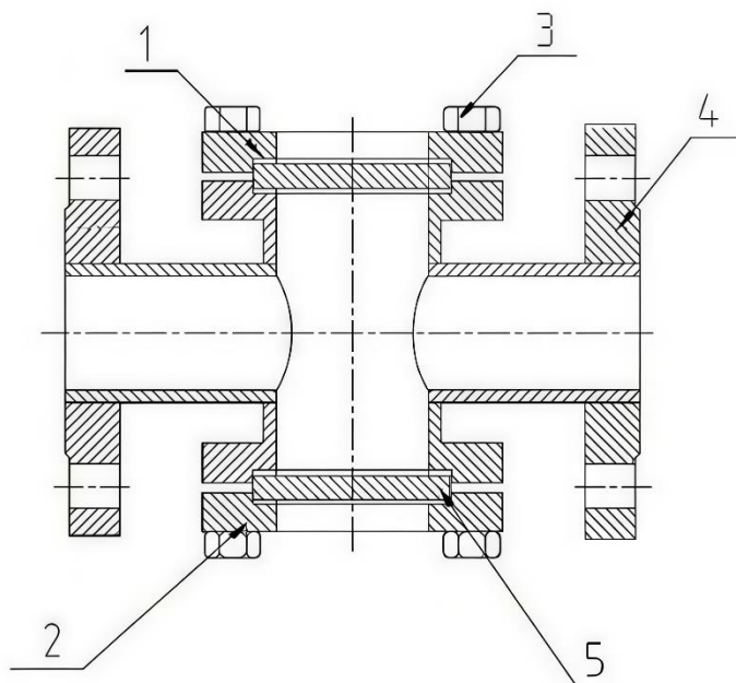
Рисунок 1 -Деталировка
