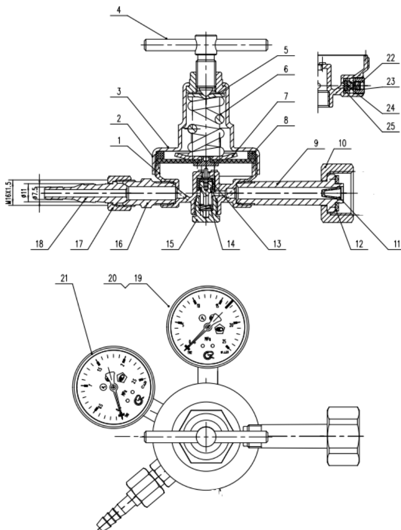
Рис. 1. Редуктор баллонный одноступенчатый
