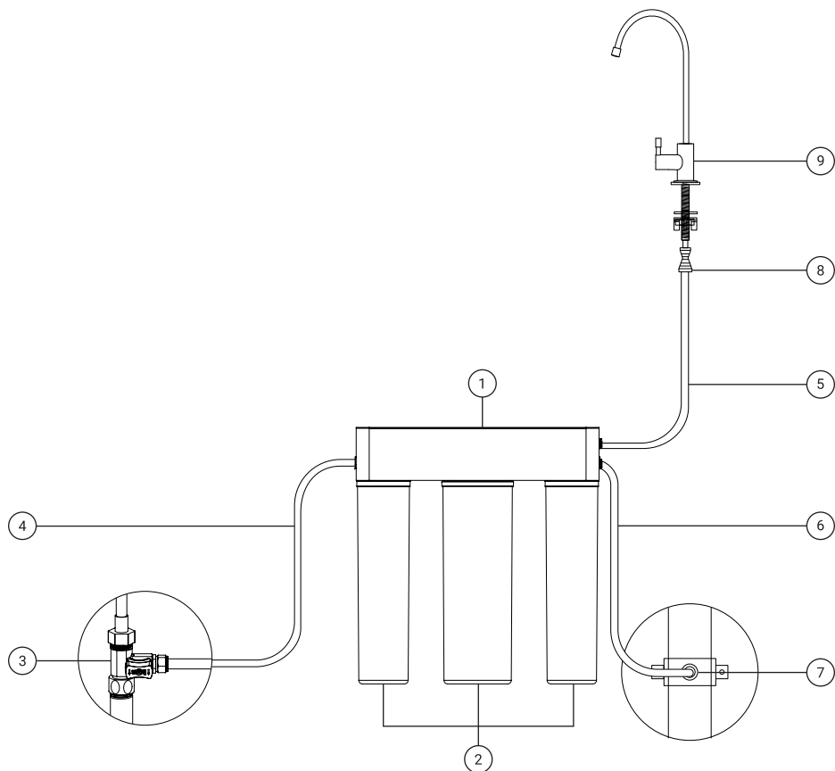
Рис. 2. Схема подключения Гейзер Прогресс
