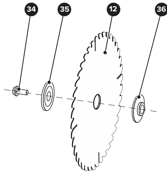
Рисунок 3 — элементы крепления пильного диска
