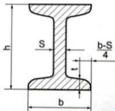
Рисунок 6. Двутавровая балка.
