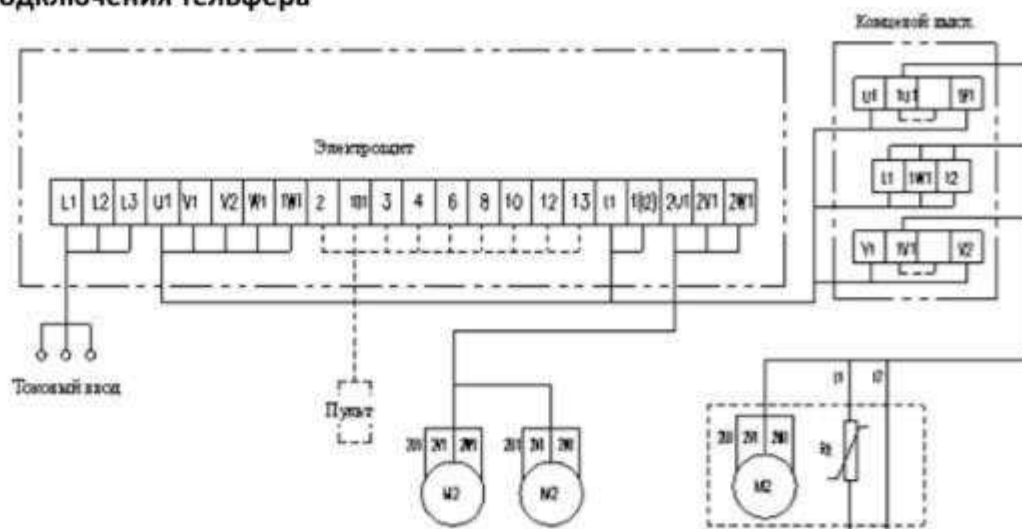
Рисунок 10. Схема подключения тельфера
