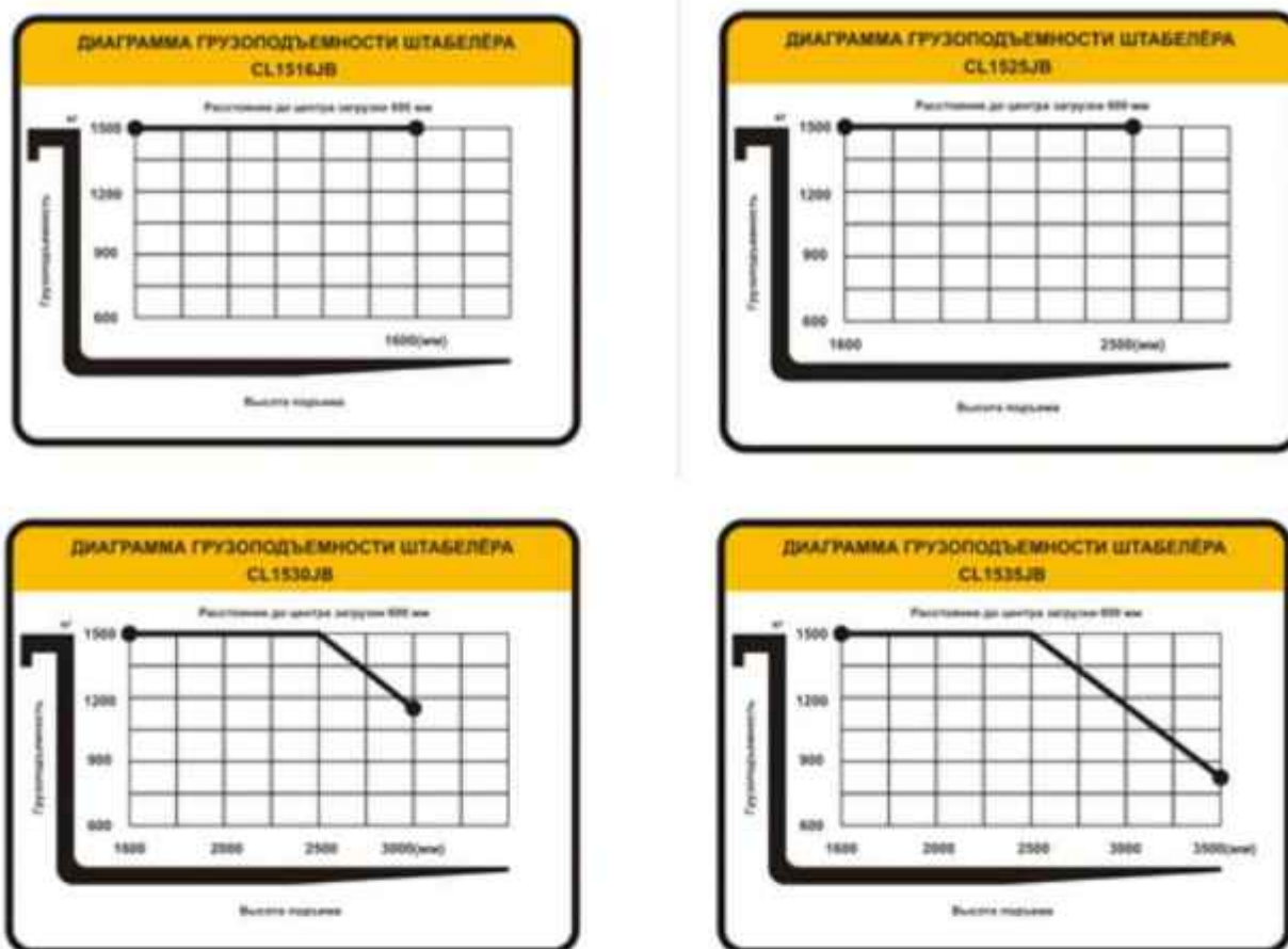
Рисунок 4. Диаграмма грузоподъемности штабелера.
