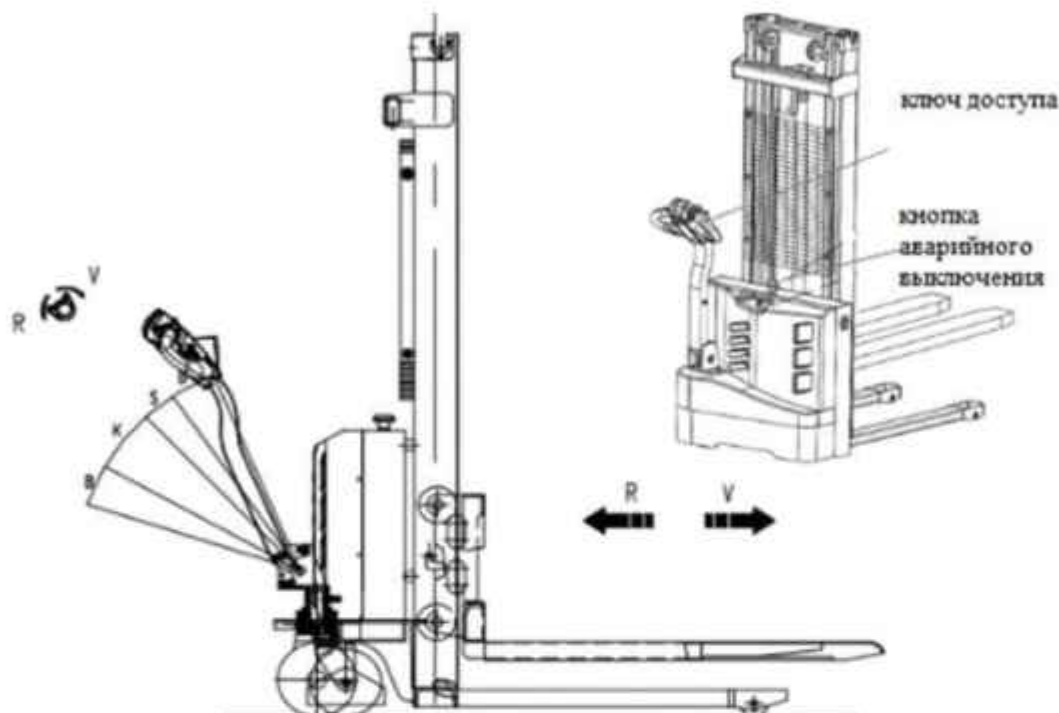
Рисунок 5. Органы управления.
