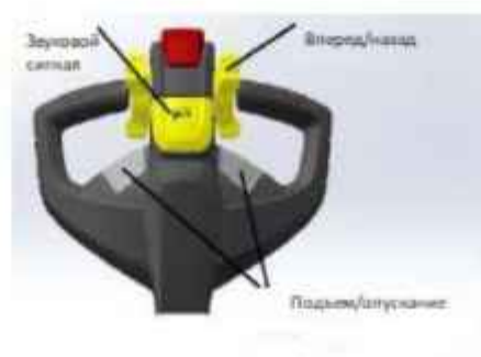
Рисунок 8. Румпель управления
